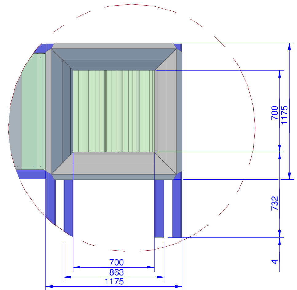
Detailansicht Anschluss Collector
