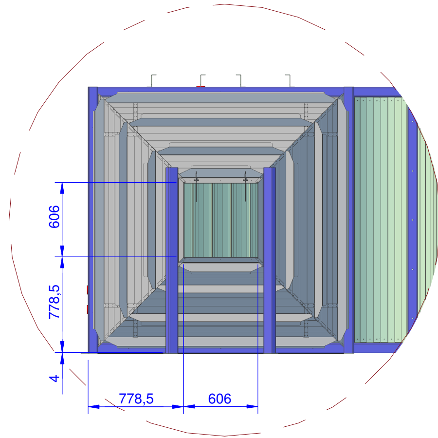
Detailansicht Anschluss Düse
